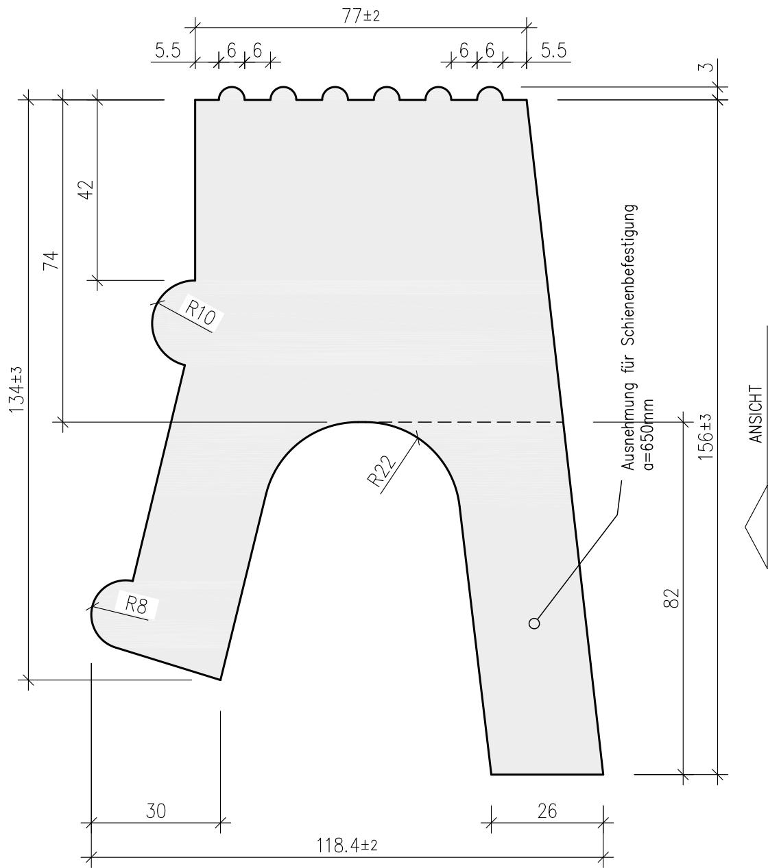
Ansicht 1:10
