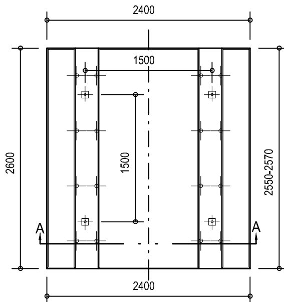
DRAUFSICHT
